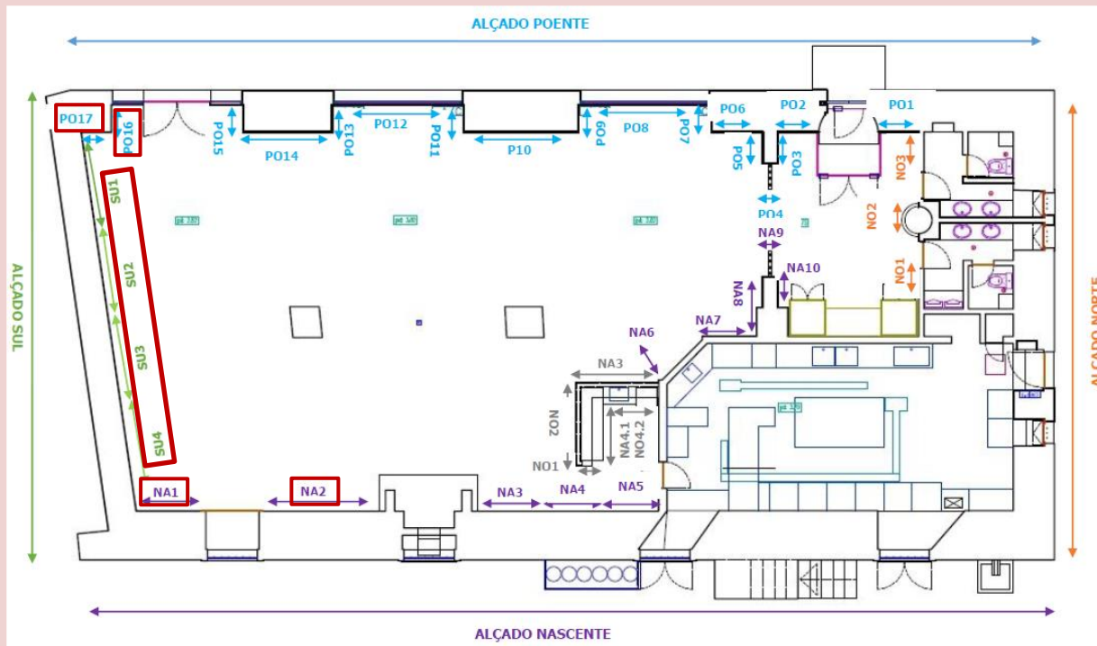
Planta interior do edifício Paço Real II (s/escala) - localização do painel PO16 PO17 SU1 SU2 SU3 SU4 NA1 NA2
