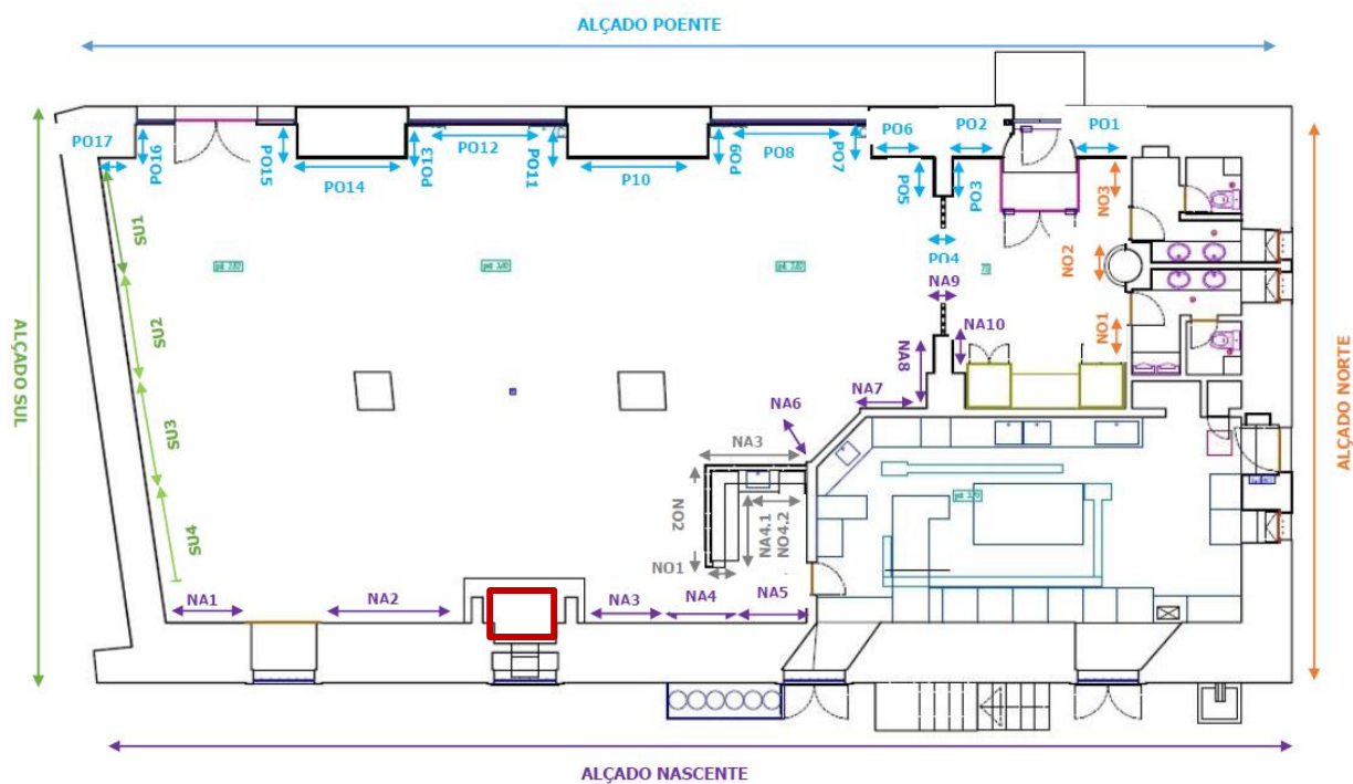
Planta interior do edifício Paço Real (s/escala) - localização da lareira no Alçado Nascente
