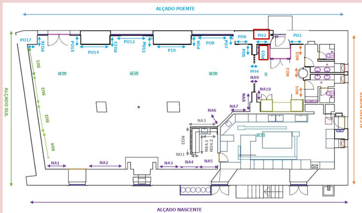
Planta interior do edifício Paço Real II (s/escala) - localização do painel: PO2 e PO3
