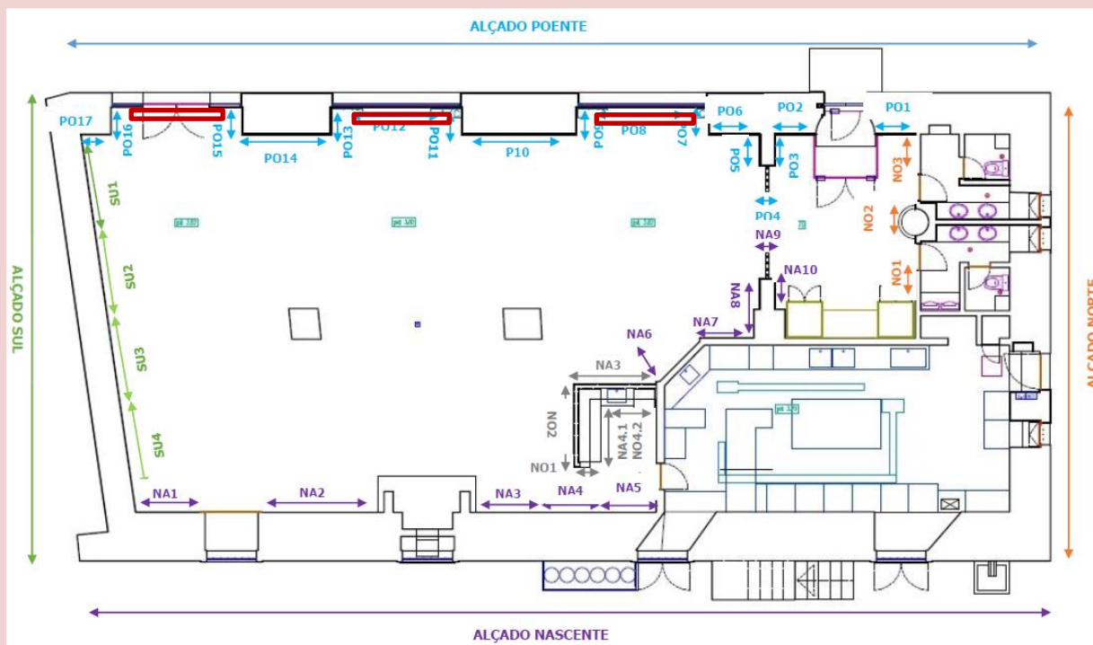
Planta interior do edifício Paço Real II (s/escala) - localização do conjunto de varões de cortinado no interior do Edifício Paço II. (Localização do património móvel aferida a 31/07/2017)
